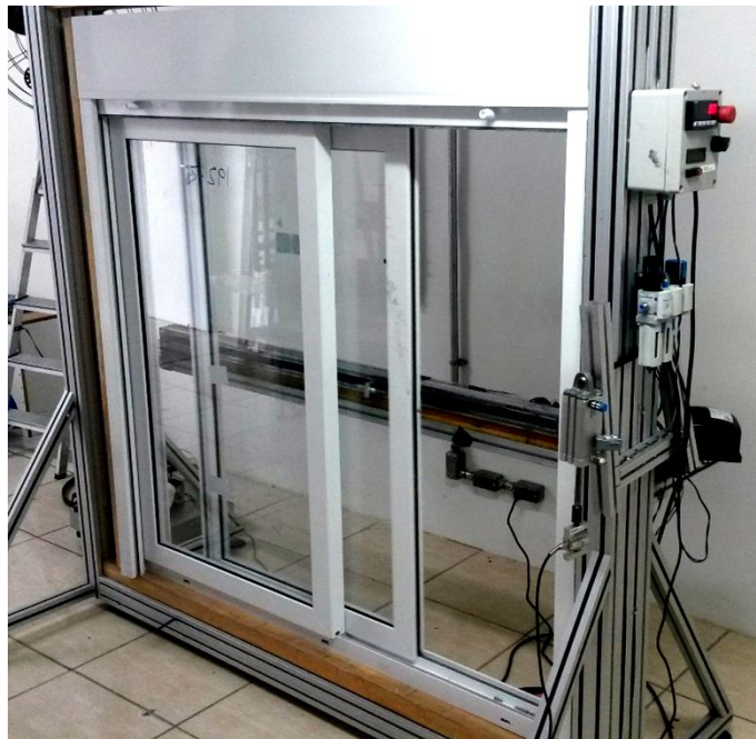
Figura 5 – Execução do ensaio de verificação do comportamento sob ações repetidas de abertura e fechamento
